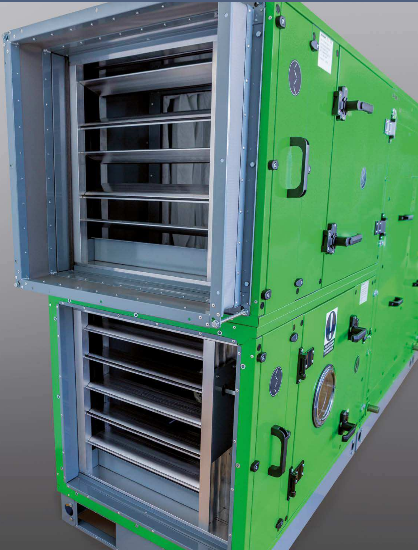
» M4 Ansicht von Ansaugseite ( oben ) und Ausblasseite ( unten )
