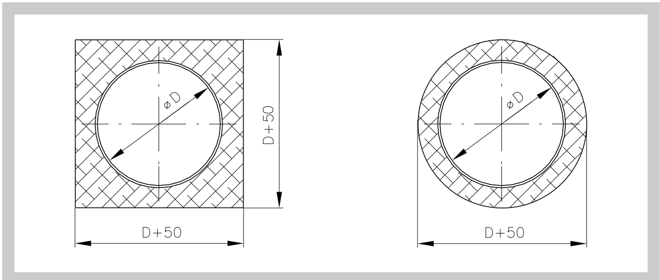
Abb. 8 Bauöffnung
