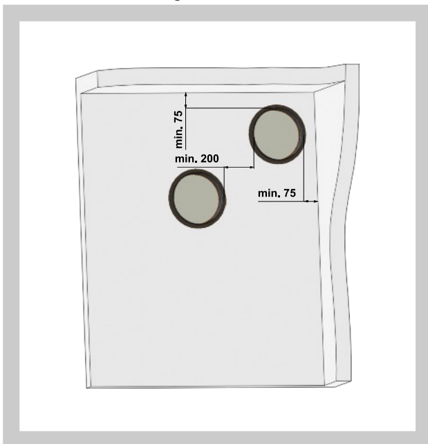
Abb. 6 Abstand zwischen den Brandschutzklappen und der Tragkonstruktion
