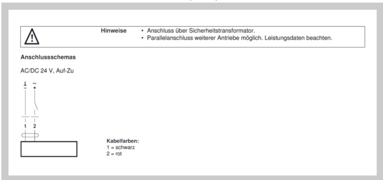
Abb. 12 Anschlussschema der Servoantriebe Belimo LF 24, NF 24A, SF 24A
