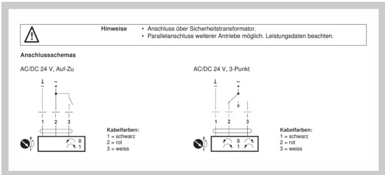
Abb. 9 Anschlussschema der Servoantriebe Belimo LM 24A-SR, NM 24A-SR, SM 24A-SR und GM 24A-SR
