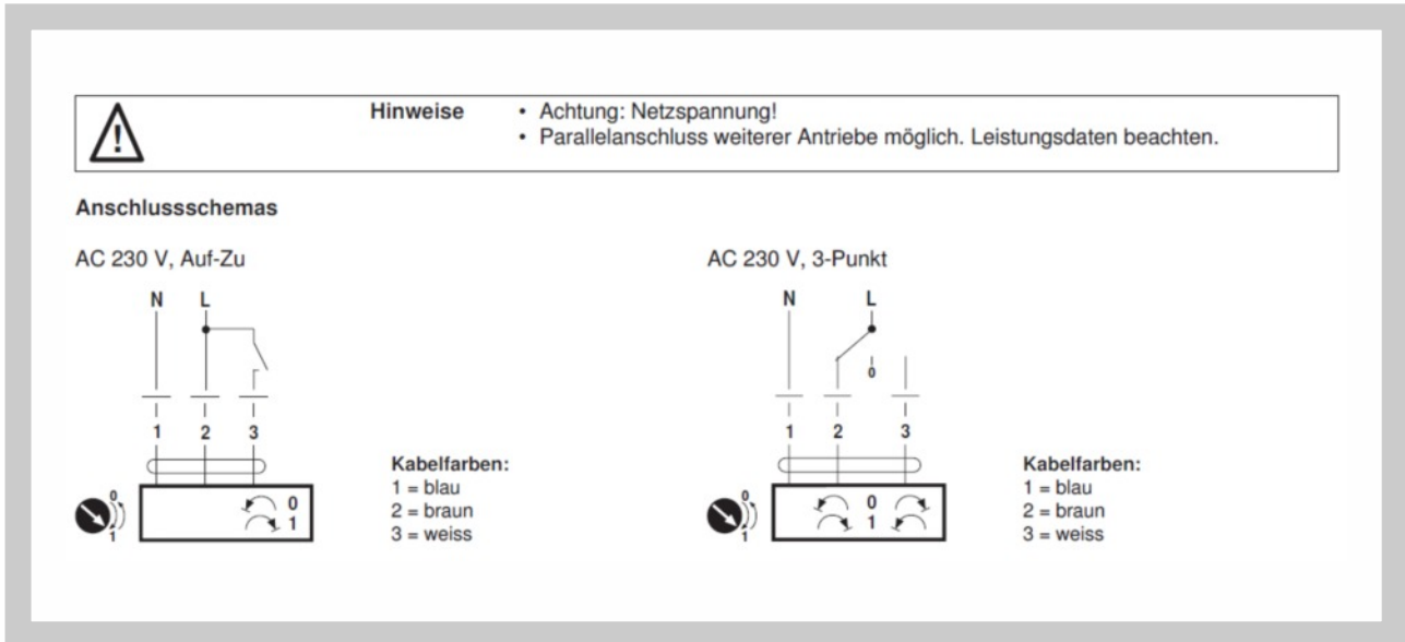
Abb. 8 Anschlussschema der Servoantriebe Belimo LM 24A, NM 24A, SM 24A und GM 24A
