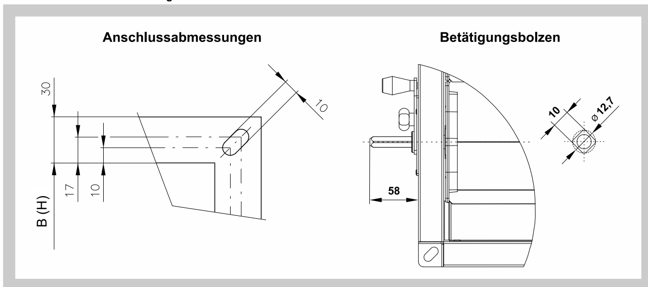
Abb. 6 Anschlussabmessungen
