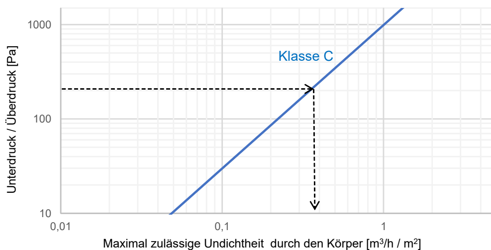
Diagramm 4 Dichtigkeit über den Körper Klasse C nach EN 1751
