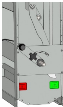
Abb. 3 Ausführung mit der Handbedienung und der Verriegelung
