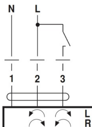
Abb. 8 Anschlussschema der Servoantriebe Belimo CM 24-L
