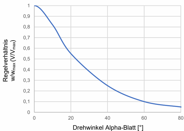
Diagramm 1 Durchflussskennlinie bei der ständigen Regeldruckdifferenz von 40 Pa
