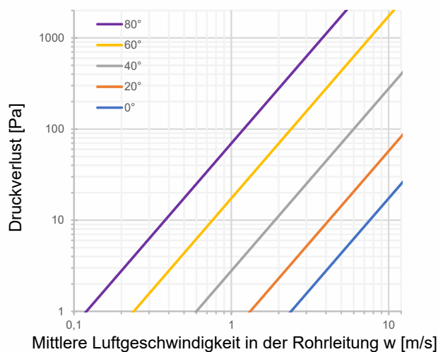
Diagramm 3 Regeldruckverlust in der Abhängigkeit vom Drehwinkel für Klappen, die Klappe am Ende der Rohrleitung
