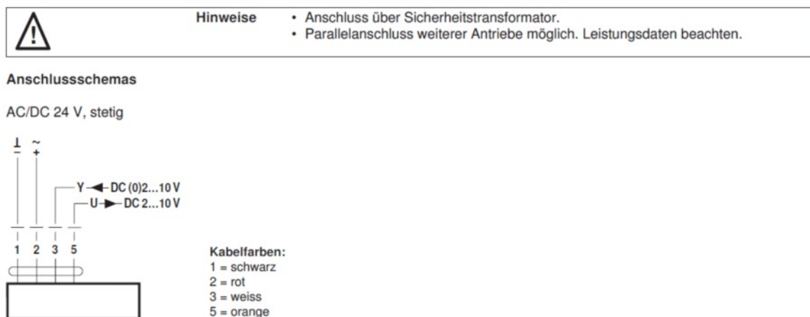
Abb. 12 Anschlussschema der Servoantriebe Belimo LM 24A-SR, NM 24A-SR und SM 24A-SR
