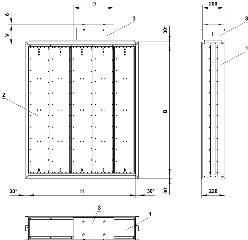
Abb. 14 Klappe SEDS-L
