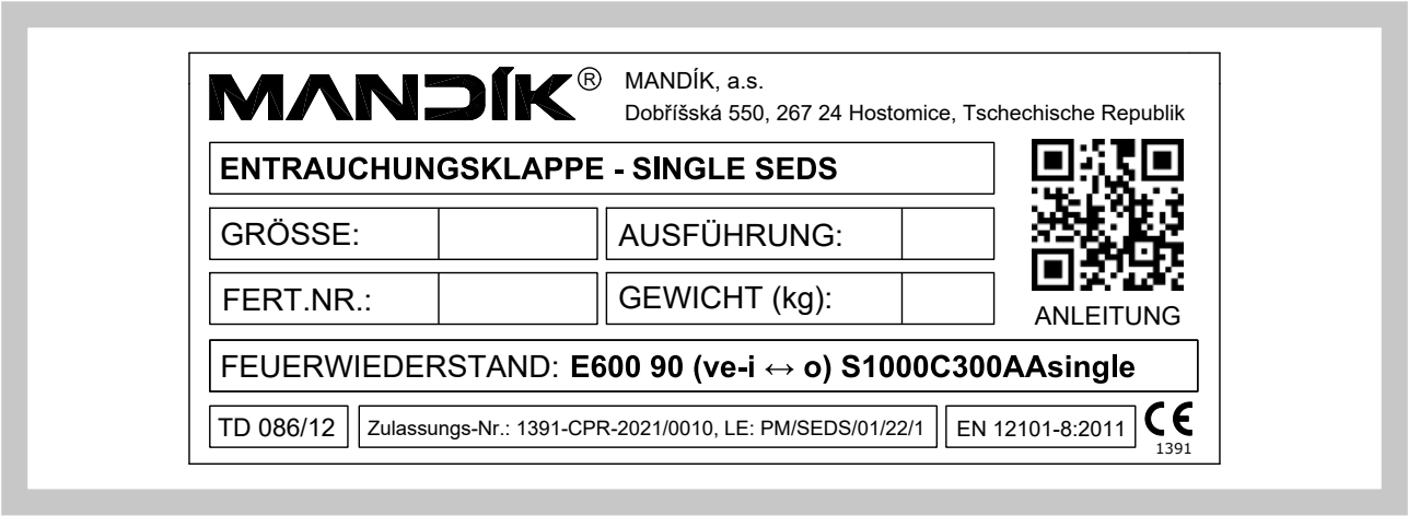
Abb. 15 Typenschild
