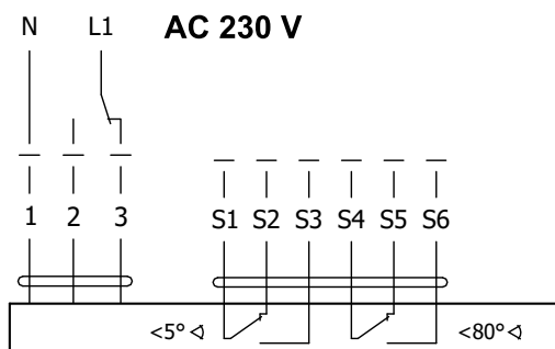
Abb. 7 Stellantrieb BELIMO BEN 230
