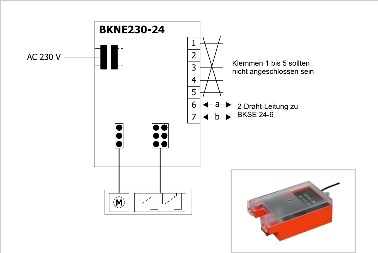
Abb. 13 Kommunikations- und Stromversorgungseinrichtung BKNE 230-24
