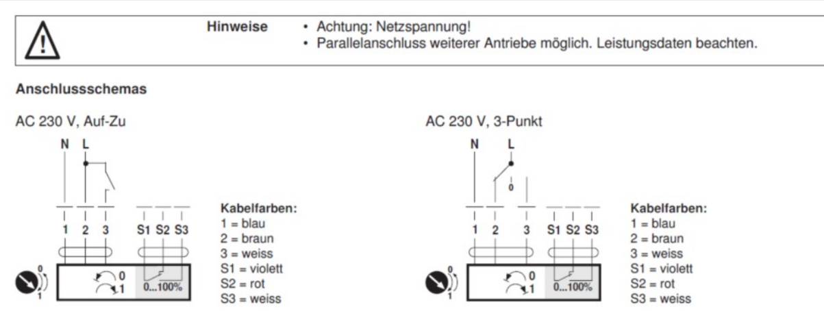
Abb. 7 Belimo LM 230A-S, NM 230A-S und SM 230A-S - Ausführung .46
