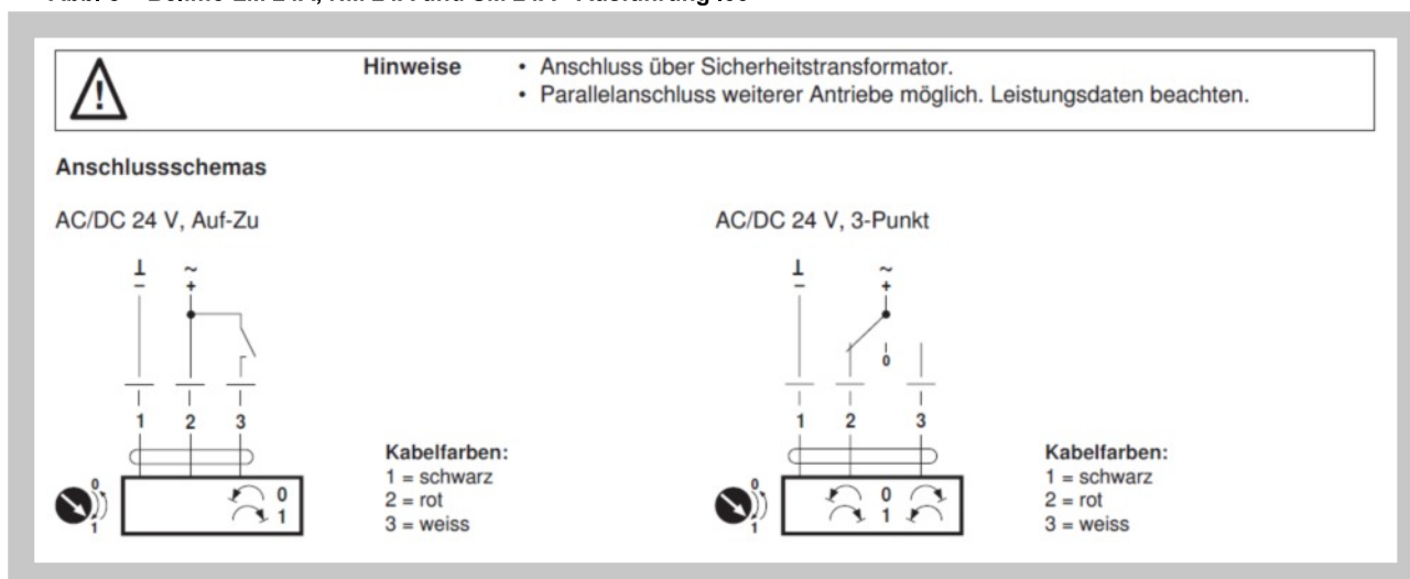
Abb. 8 Belimo LM 24A, NM 24A und SM 24A - Ausführung .55
