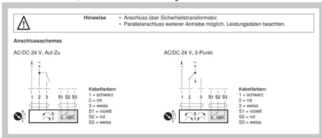
Abb. 9 Belimo LM 24A-S, NM 24A-S und SM 24A-S - Ausführung .56
