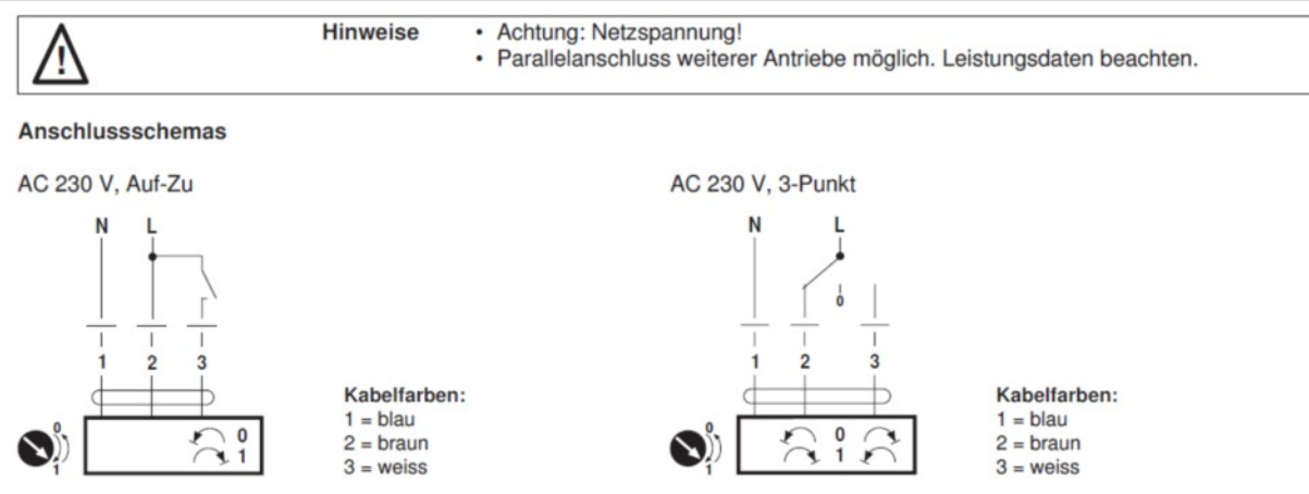
Abb. 6 Belimo LM 230A, NM 230A und SM 230A - Ausführung .45
