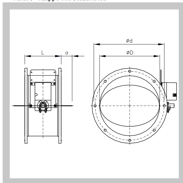
Abb. 3 Klappe mit Stellantrieb
