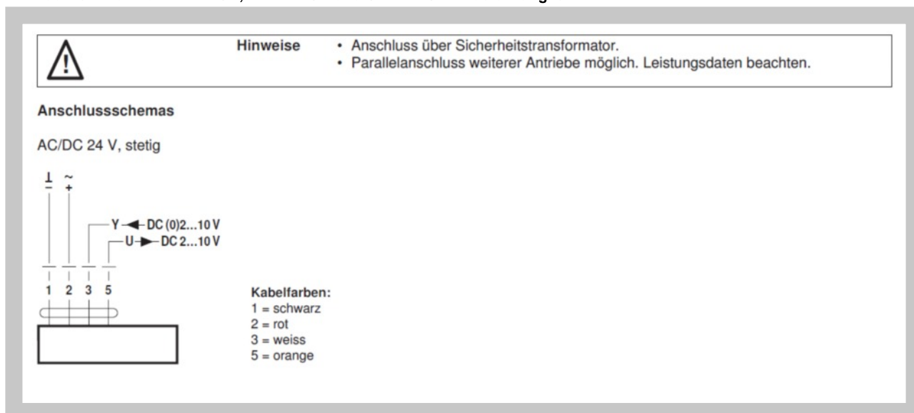
Abb. 10 Belimo LM 24A-SR, NM 24A-SR und SM 24A-SR - Ausführung .57
